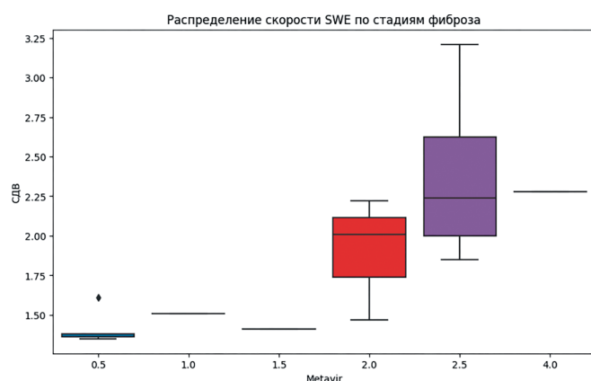
Рис. 3. По оси X отложены степени фиброза по результатам биопсии, по оси Y — скорости сдвиговых волн. Видно, что наибольший разброс получается, когда стадия по биопсии соответствует F2 и F2–F3
