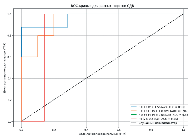
Рис. 2. ROC-анализ. Представлены кривые для порогов F \geq F2 , F \geq F2-F3 , F \geq F3-F4 и F=F4 , а также кривая случайного классификатора
